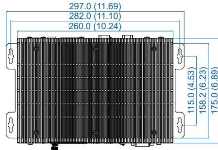
ECX-2000F-2G
