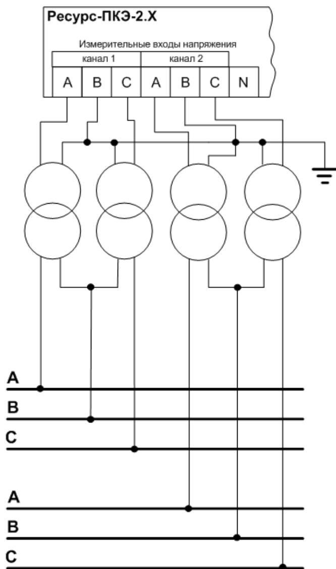
а) два фидера
