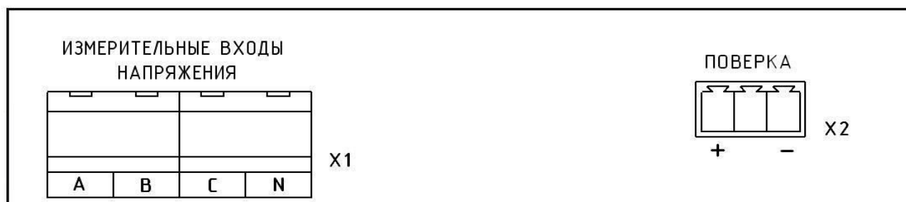
Рисунок Б.6 – Расположение элементов измерительного клеммного отсека приборов «Ресурс-ПКЭ-1.Х-ои-Х»
