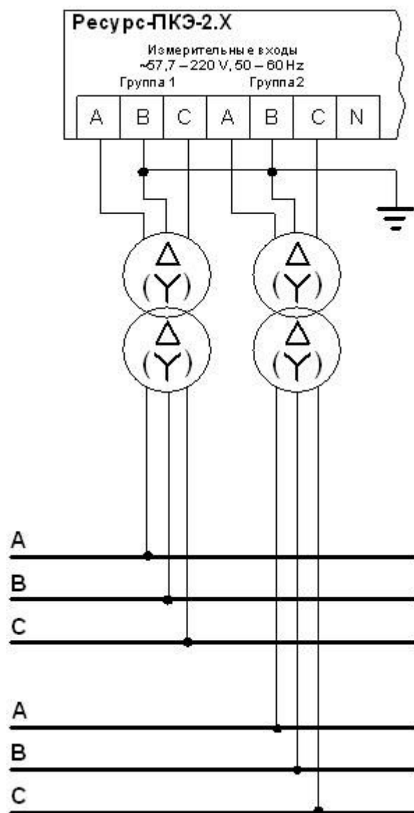
а) два фидера
