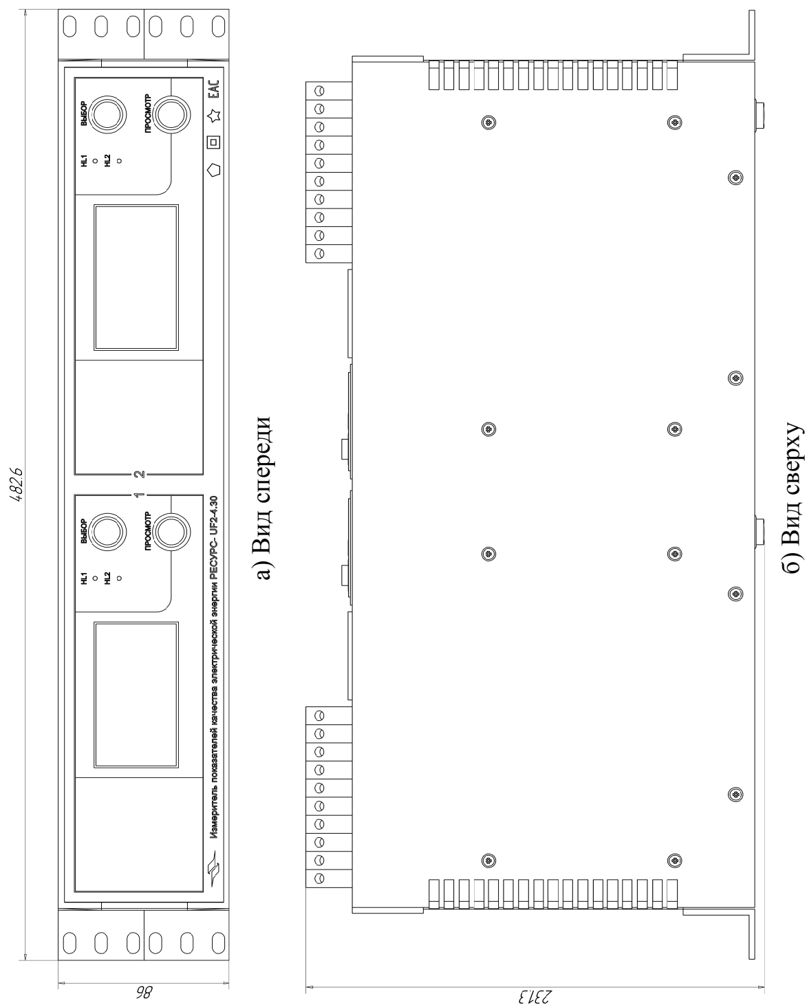
Рисунок А.7 – Габаритные размеры приборов «Ресурс-UF2-4.30-X-X-c-XXX» и «Ресурс-UF2-4.30-X-X-2c-XXX»
