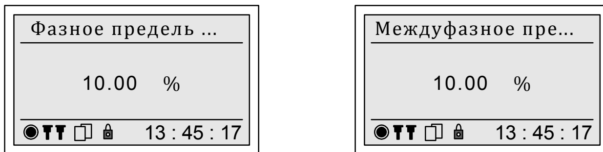
Рисунок 58 – Отображение предельно допустимых значений отклонений фазного и междуфазного напряжения для положительного и отрицательного отклонений напряжения
