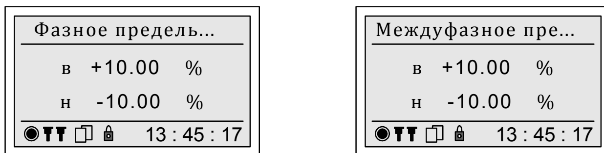
Рисунок 57 – Отображение предельно допустимых значений отклонений фазного и междуфазного напряжения для отклонения среднеквадратического значения напряжения и отклонения напряжения основной частоты
