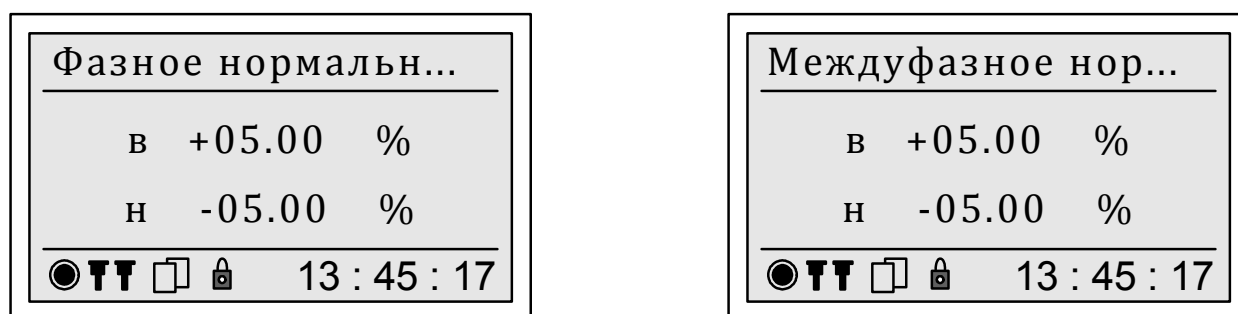
Рисунок 55 – Отображение нормально допустимых значений отклонений фазного и междуфазного напряжения для отклонения среднеквадратического значения напряжения и отклонения напряжения основной частоты
