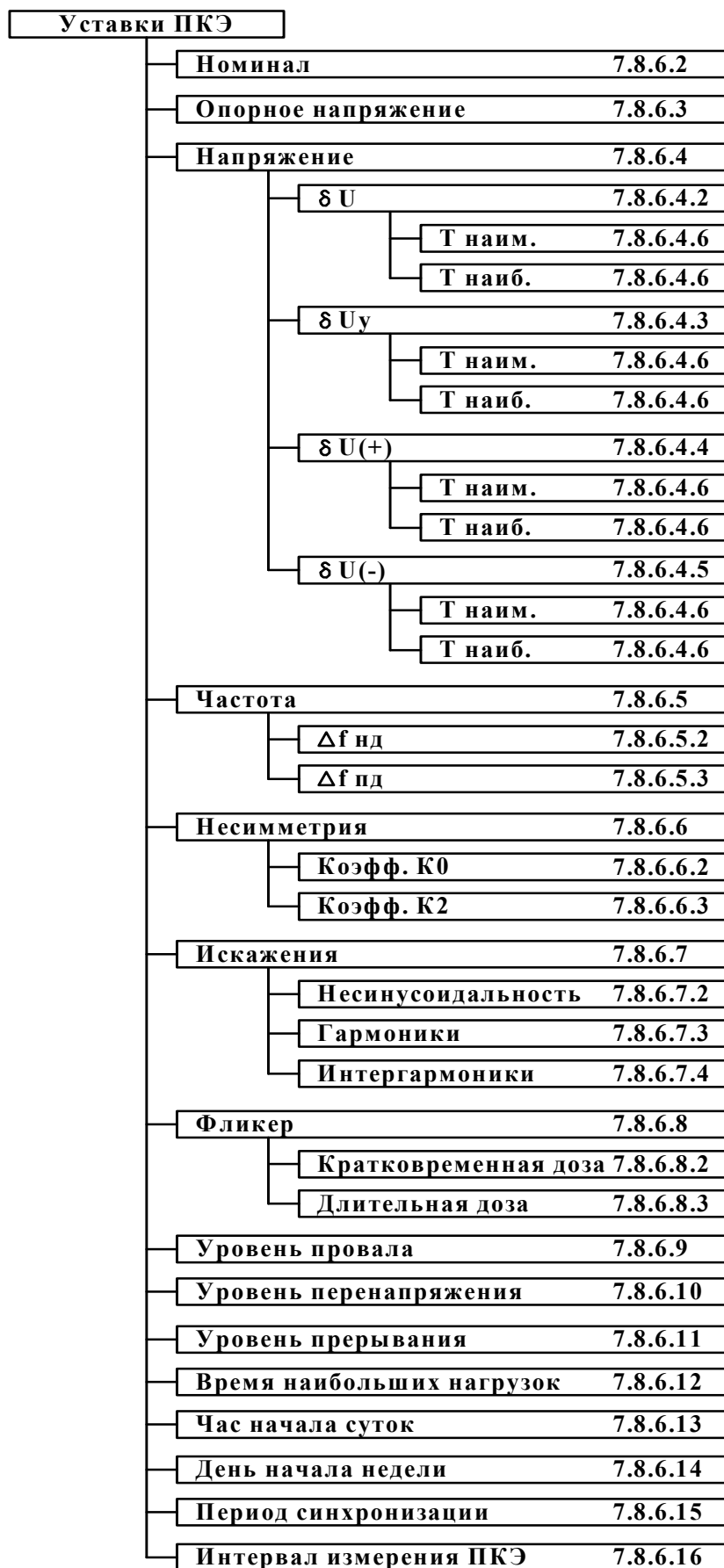
Рисунок 53 – Структура меню «Уставки ПКЭ»
