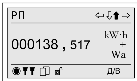
Рисунок 21 – Пример вывода результатов измерений активной энергии за расчётный период
