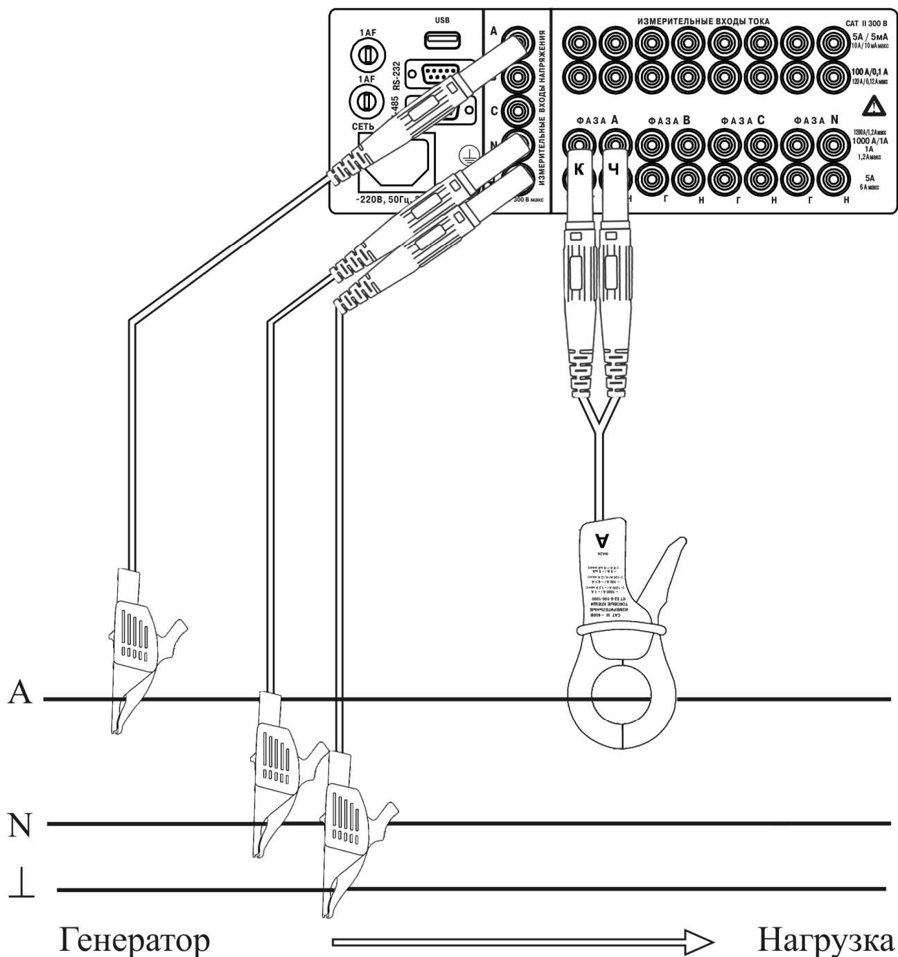
Рисунок Р.5 – Схема подключений прибора модификации «Ресурс–UF2M-3T52-5-100-1000» для измерений в однофазной трехпроводной системе с помощью токоизмерительных клещей КТ52-5-100-1000 на пределе 1000 А
