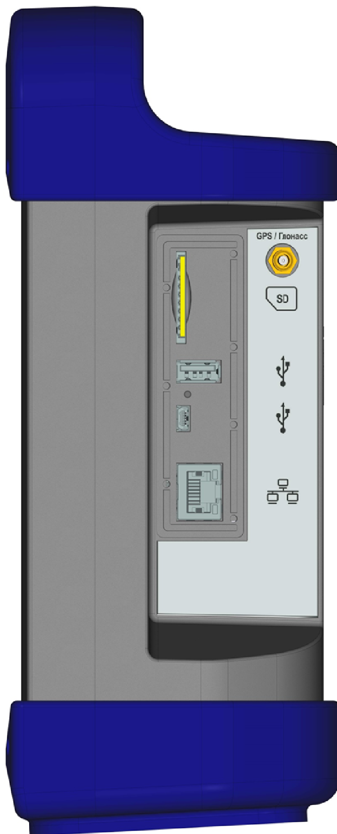
Рисунок А.3 – Внешний вид справа приборов «Ресурс-PQA-M»
