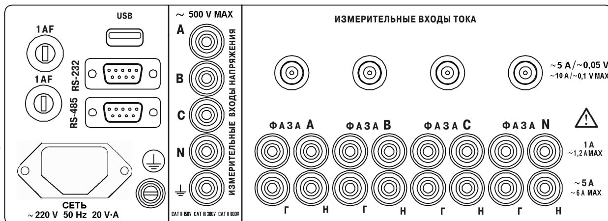
Рисунок П.1 – Задняя панель прибора модификаций «Ресурс–UF2М-3П15-5» и «Ресурс–UF2М-4П15-5»
