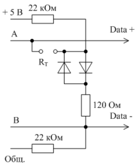
а) Выходной каскад интерфейса RS-485 «Ресурс–UF2»
