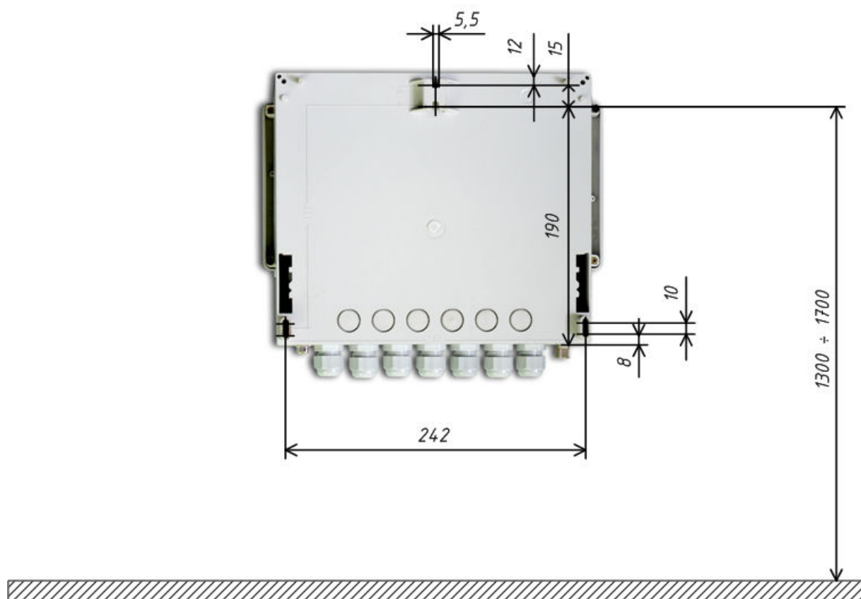
Рисунок Д.1 – Габаритные размеры прибора модификаций «Ресурс–UF2» и «Ресурс–UF2С»
