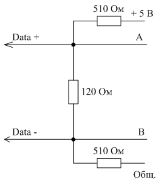
б) Выходной каскад ведущего устройства
