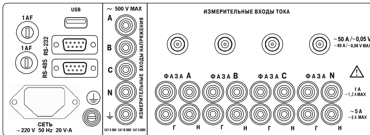
Рисунок П.2 – Задняя панель прибора модификаций «Ресурс–UF2М-3П15-50» и «Ресурс–UF2М-4П15-50»
