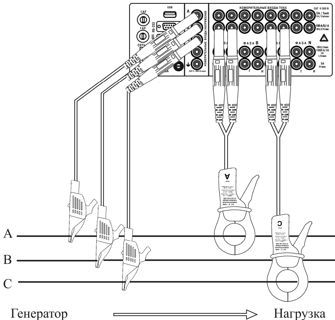
Рисунок Р.3 – Схема подключений прибора модификации «Ресурс–UF2M-3T52-5-100-1000» для измерений в трехфазной трехпроводной системе с помощью токоизмерительных клещей KT52-5-100-1000 на пределе 100 А
