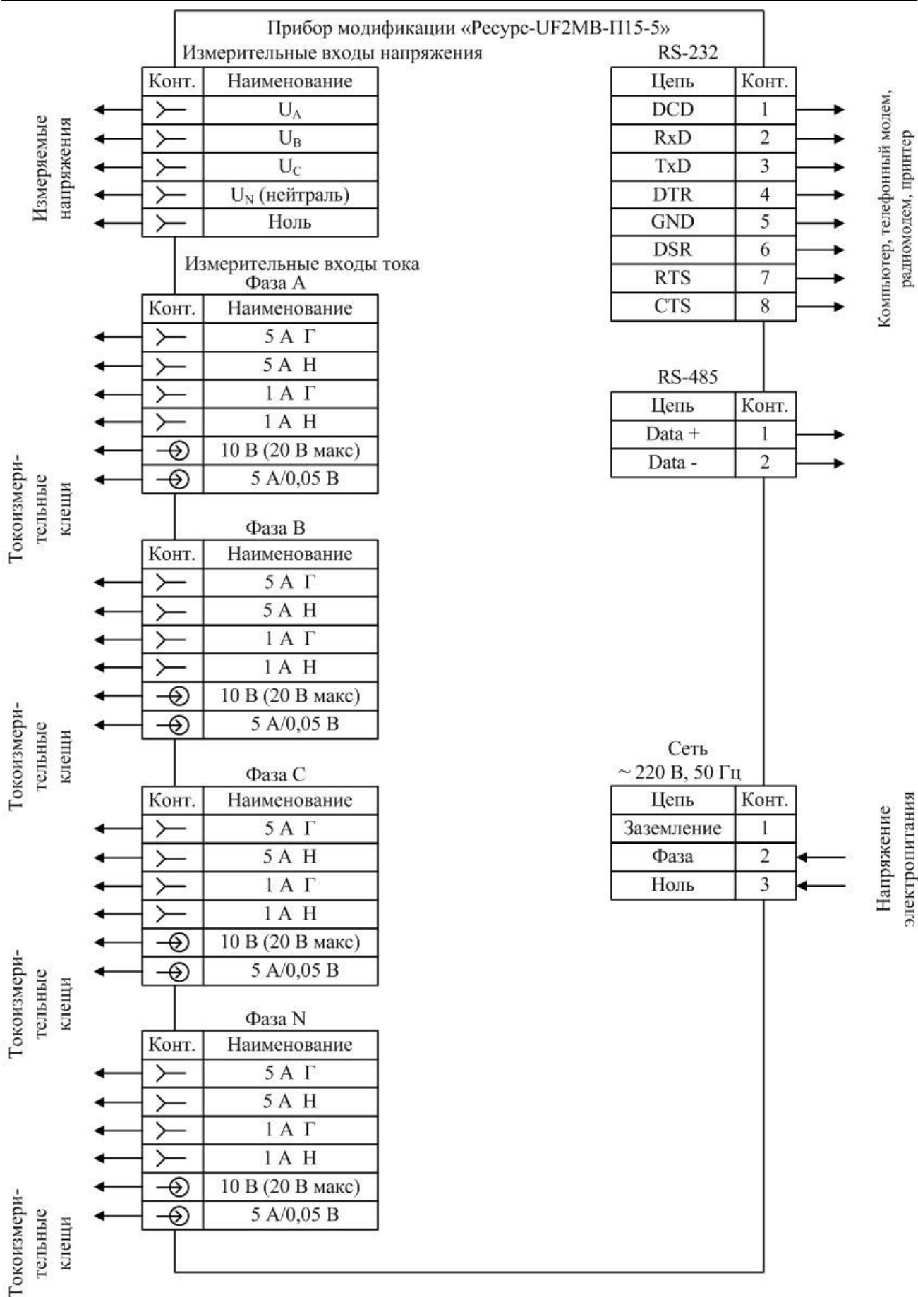
Рисунок Ж.8 – Назначение контактов разъемов прибора модификации «Ресурс–UF2MB-П15-5»
