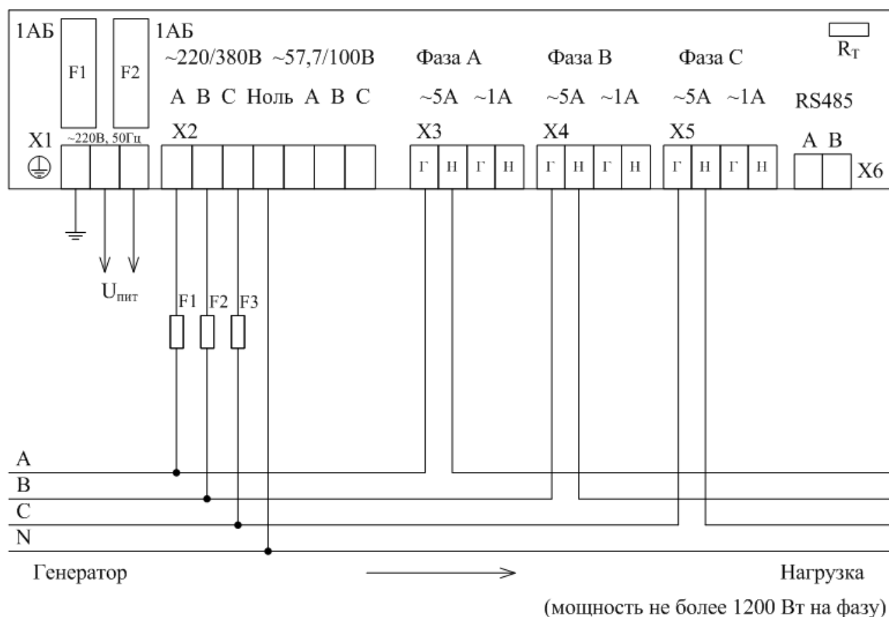
Рисунок И.5 – Трехфазная четырехпроводная схема подключений при измерении напряжения и силы тока (номинальные значения напряжения 220/380 В и тока 5 А)
