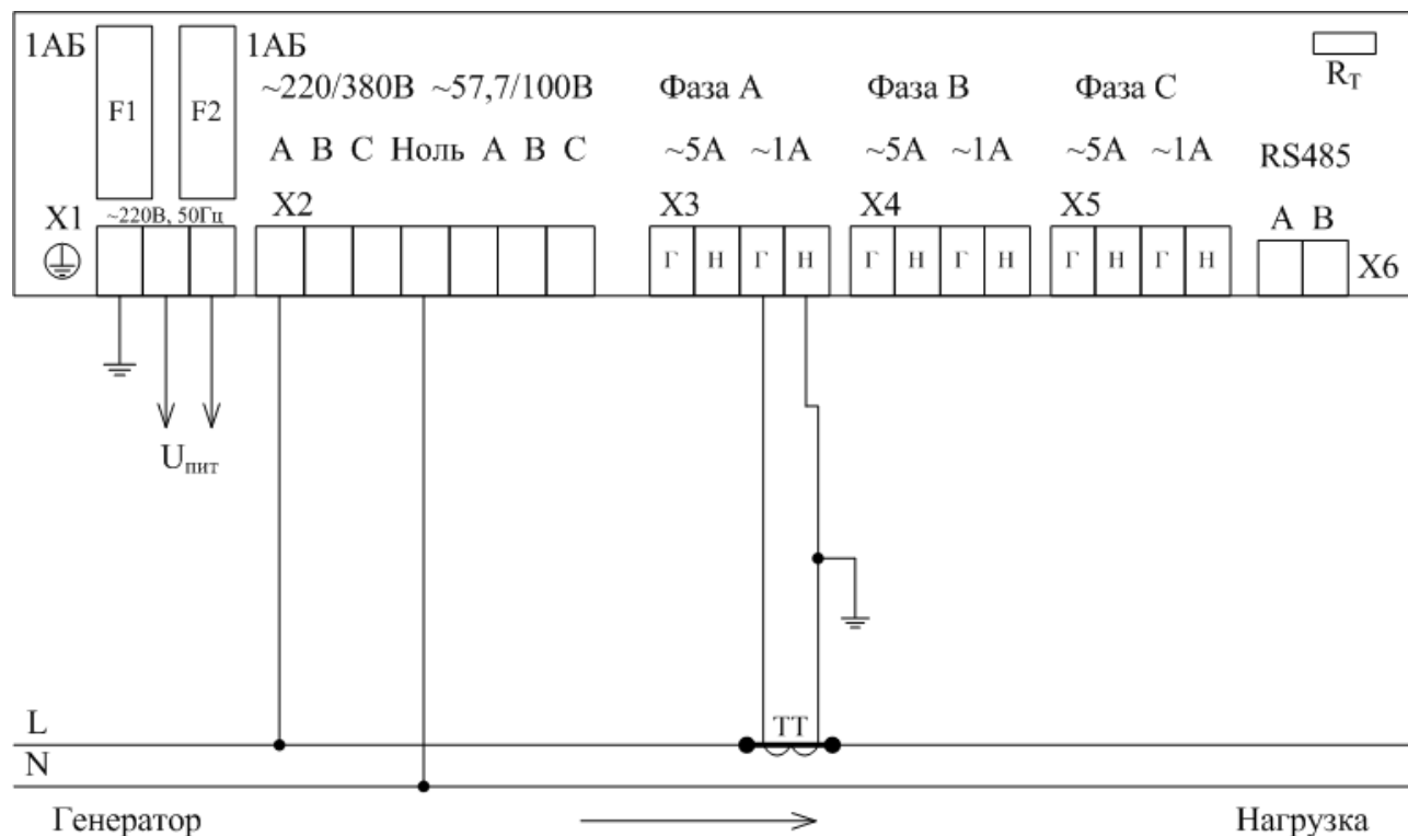
Рисунок И.4 – Однофазная схема подключений при измерении без ТН с ТТ (номинальные значения напряжения 220/380 В и тока 1 А)
