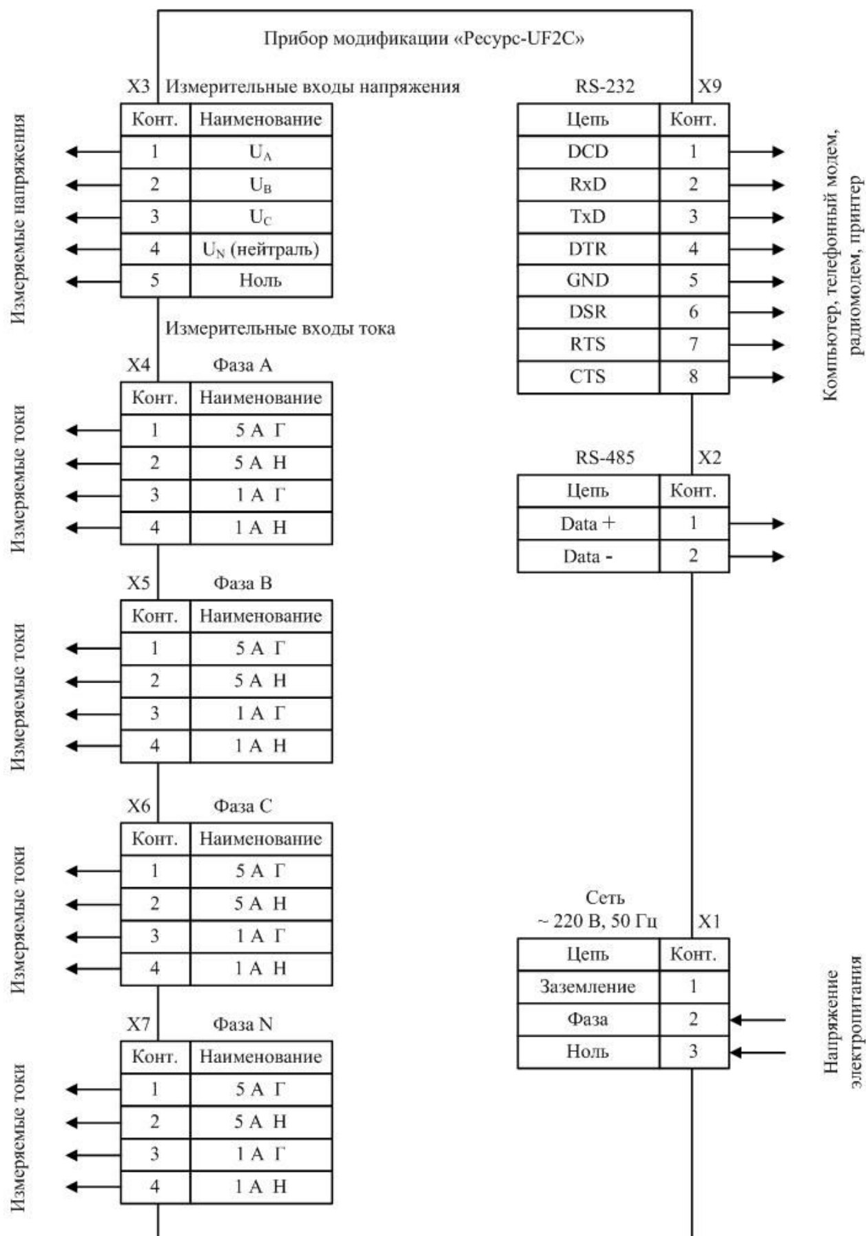
Рисунок Ж.4 – Назначение контактов разъемов прибора модификации «Ресурс–UF2C»
