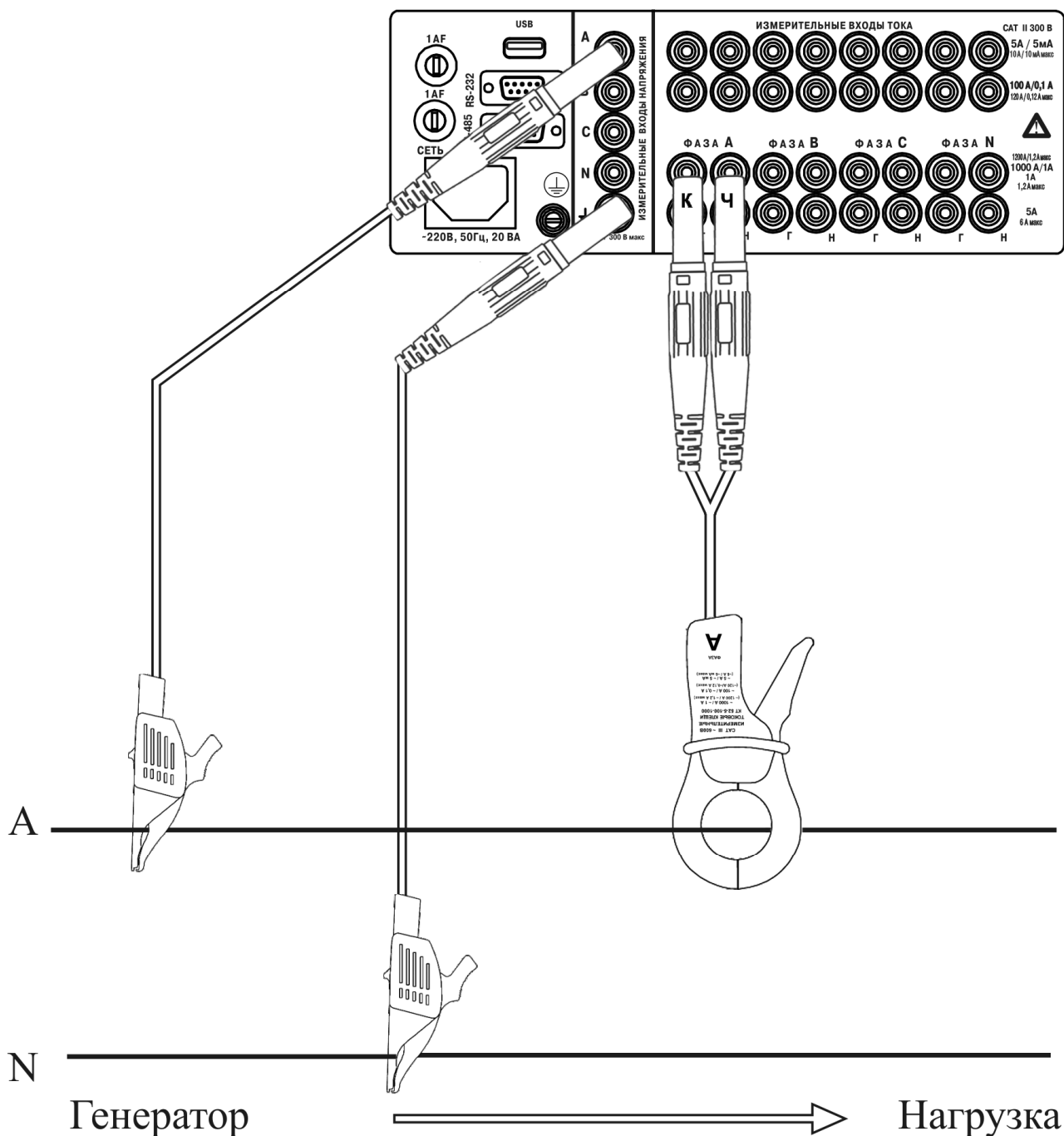
Рисунок Р.4 – Схема подключений прибора модификации «Ресурс–UF2М-3Т52-5-100-1000» для измерений в однофазной двухпроводной системе с помощью токоизмерительных клещей KT52-5-100-1000 на пределе 1000 А
