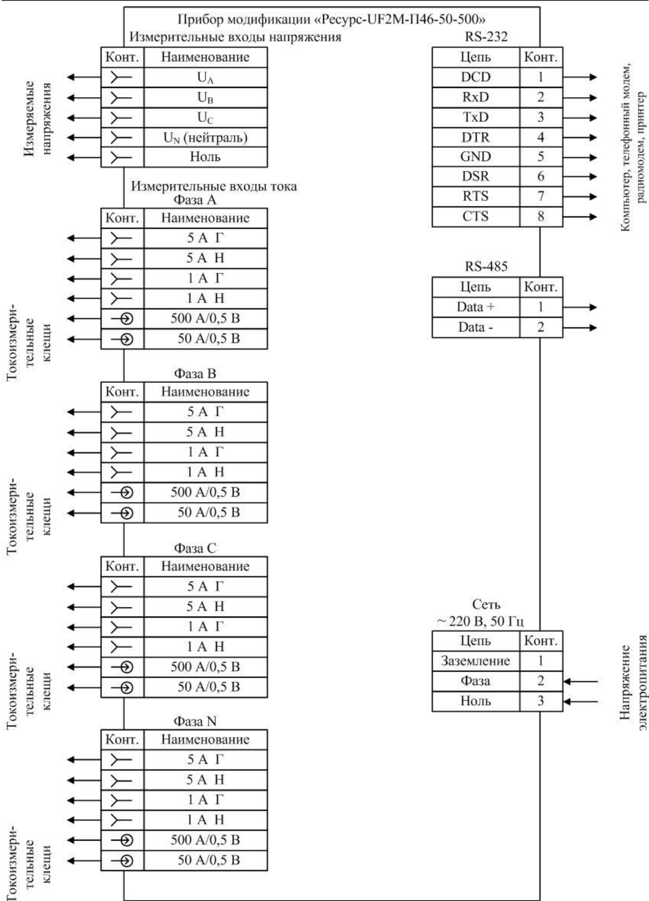
Рисунок Ж.7 – Назначение контактов разъемов прибора модификации «Ресурс–UF2М-П46-50-500»
