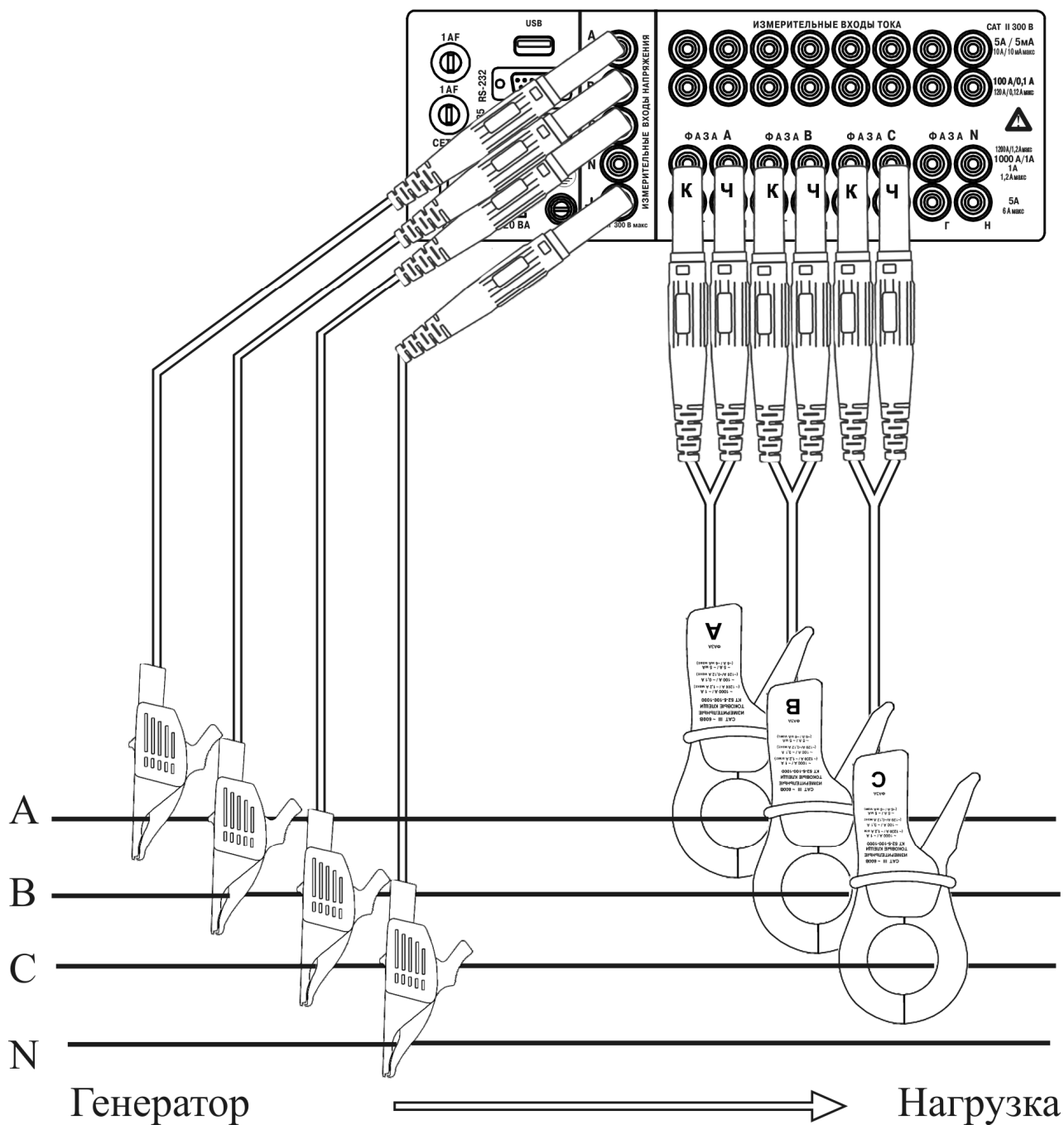
Рисунок Р.2 – Схема подключений прибора модификации «Ресурс–UF2M-3T52-5-100-1000» для измерений в трехфазной четырёхпроводной системе с помощью токоизмерительных клещей KT52-5-100-1000 на пределе 1000 А
